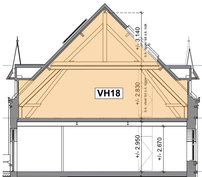
Doorsnede A-A
