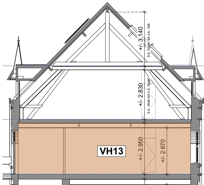
Doorsnede A-A
