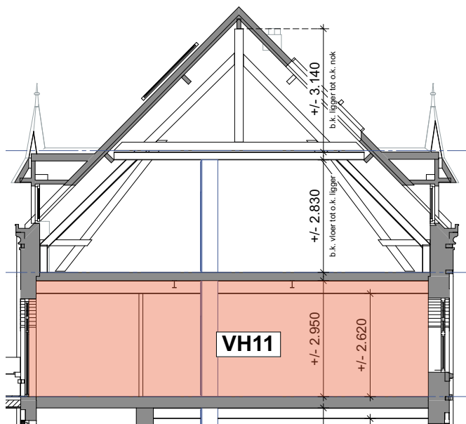
Doorsnede A-A
