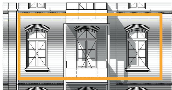
Achtergevel
