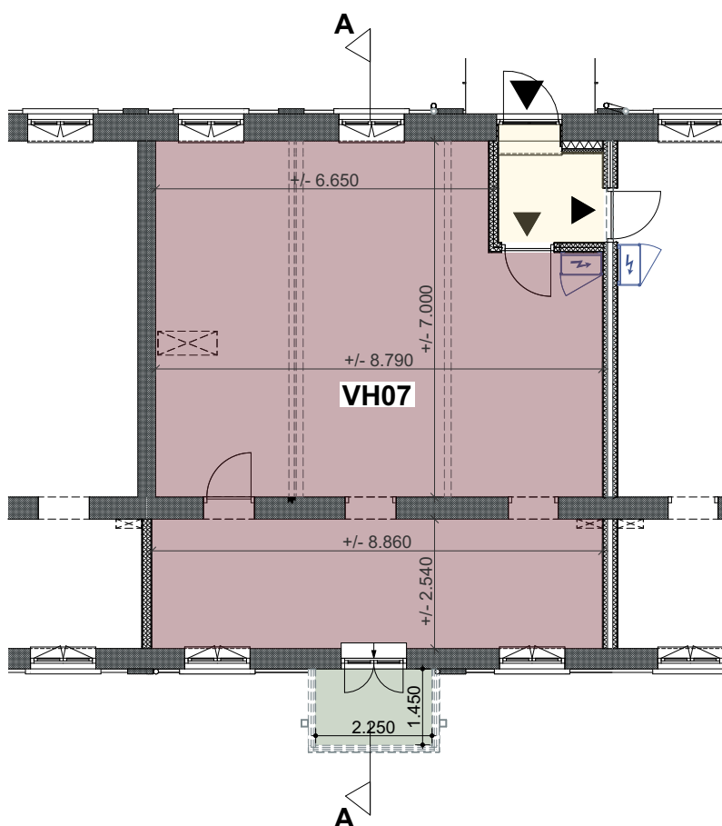
Eerste verdieping
