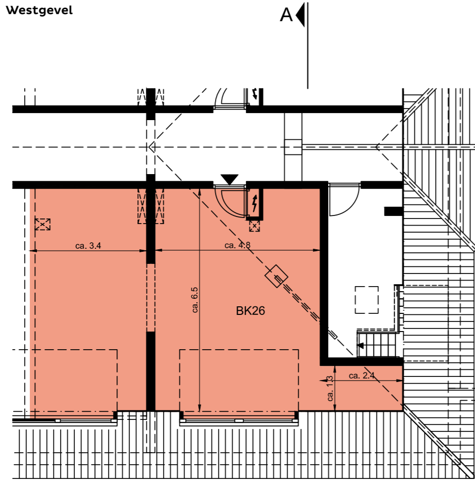
Begane grond
