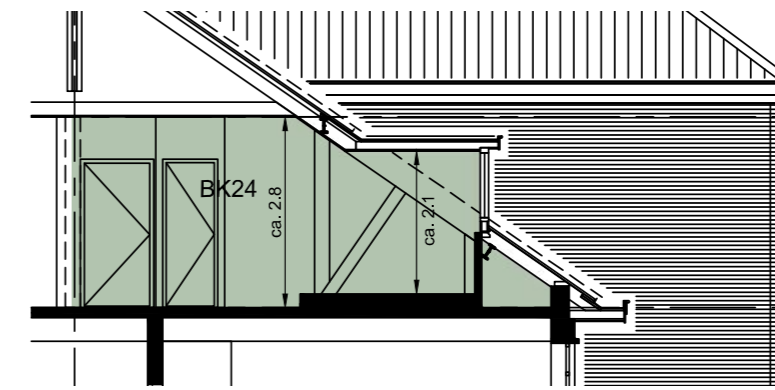
Doorsnede A-A
