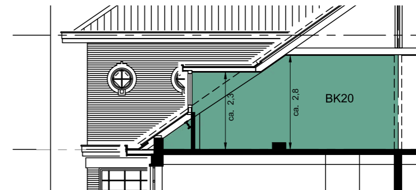
Doorsnede A-A
