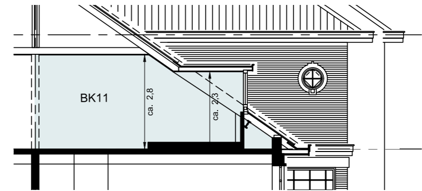
Doorsnede A-A
